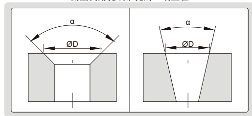
测量倒角孔或锥孔的口端直径
